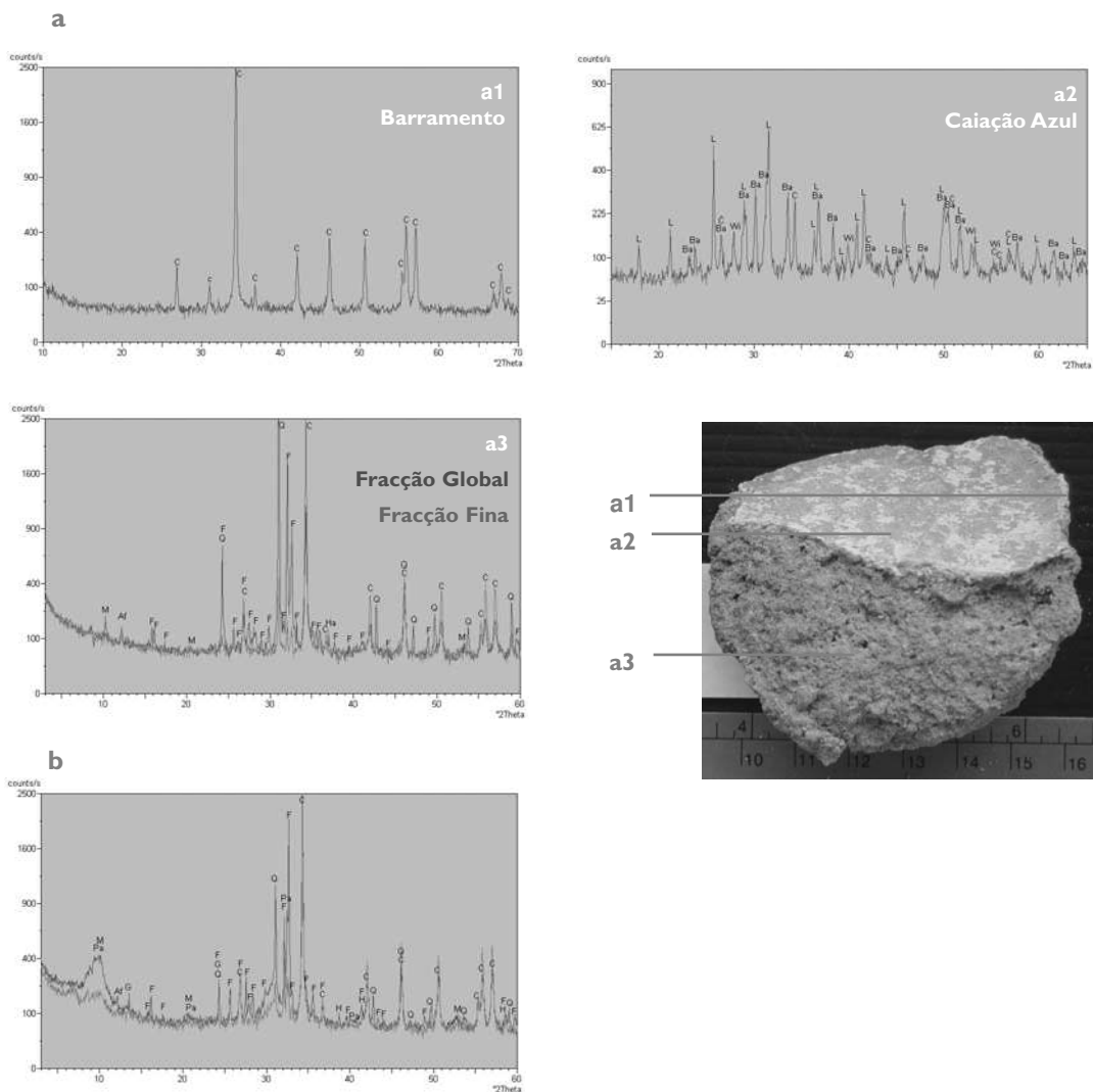
Fig. 6 Difractogramas de raios X das amostras estudadas: a) amostra VA5; b) amostra VA6. Símbolos: Af - anfíbola; Ba - barita ( BaSO_4 ); C - calcite ( CaCO_3 ); F - feldspato; G - gesso ( CaSO_4 ); H - hematite ( Fe_2O_3 ); Ha - Halite ( NaCl ); L - laurionite ( PbClOH ); M - mica; Pa - paligorsquite; Q - quartzo ( SiO_2 ); Wi - witherite ( BaCO_3 ).
