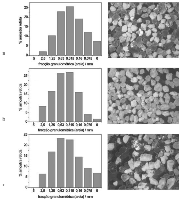
Fig. 4 Distribuições de tamanho de partículas das areias e fotografias à lupa binocular do resíduo insolúvel correspondentes à fracção entre 1,25 mm e 0,65mm: a) amostra VA3; b) amostra VA5; c) amostra VA6.
