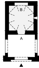
Planta, piso térreo
