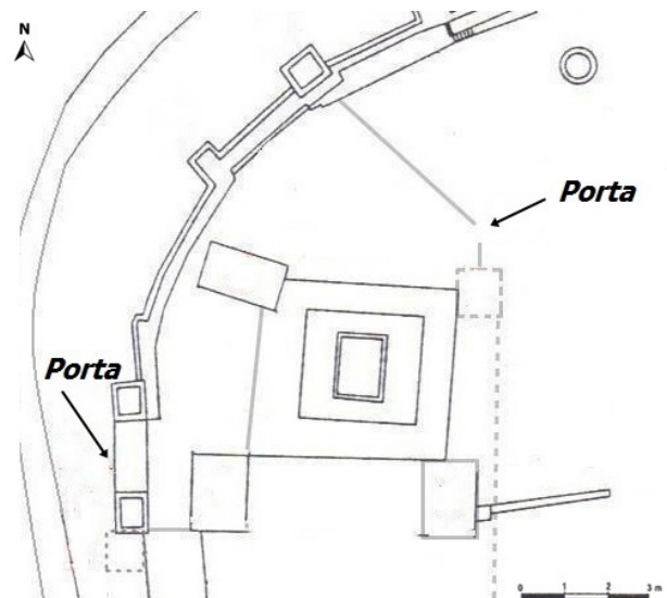
Fig. 5 - Planta da alcáçova (cedida pelo Gabinete de Arqueologia da Câmara Municipal de Alcácer do Sal/modificada pela autora).
